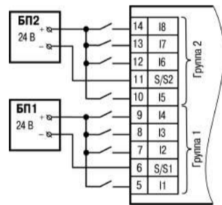
Рисунок 4 – Схема подключения дискретных датчиков с выходом типа «сухой контакт»
