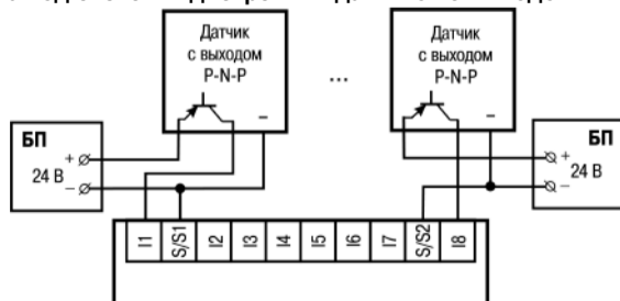
Рисунок 5 – Схема подключения трехпроводных дискретных датчиков, имеющих выходной транзистор р-п-р-типа с открытым коллектором
