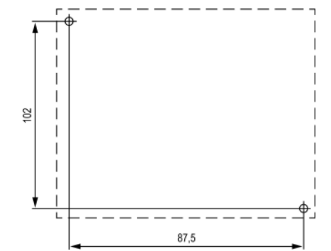
Рисунок 2 – Разметка для монтажа на стену
