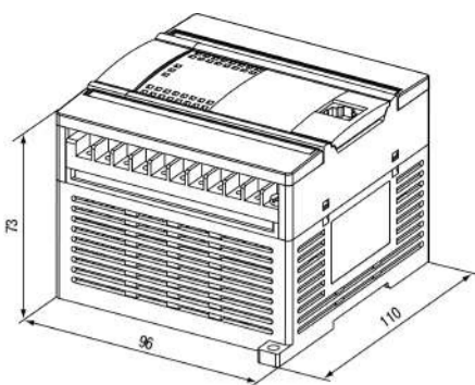
Рисунок 1 – Габаритный чертёж
